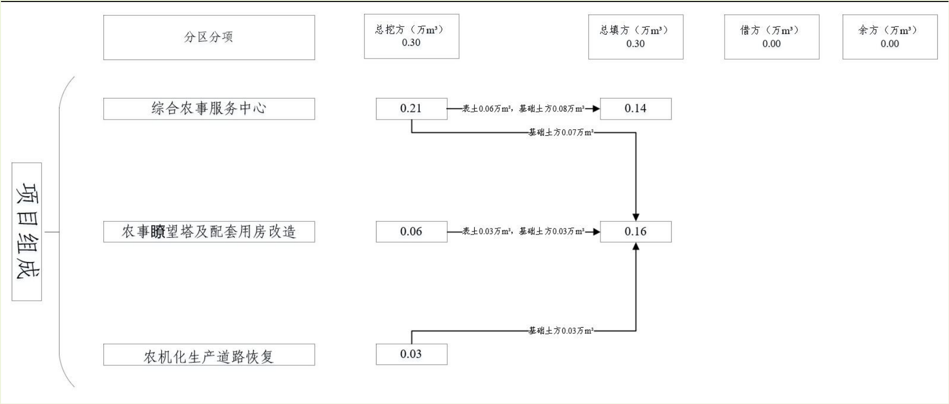
图 2.4-1 土石方流向框图 单位万 m³ (自然方)
